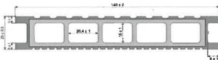
Rys. 3. Deska tarasowa WPC GAMRAT 140x25 dwustronnie ryflowana
