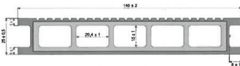
Rys. 2. Deska tarasowa WPC GAMRAT 140x25 jednostronnie ryflowana
