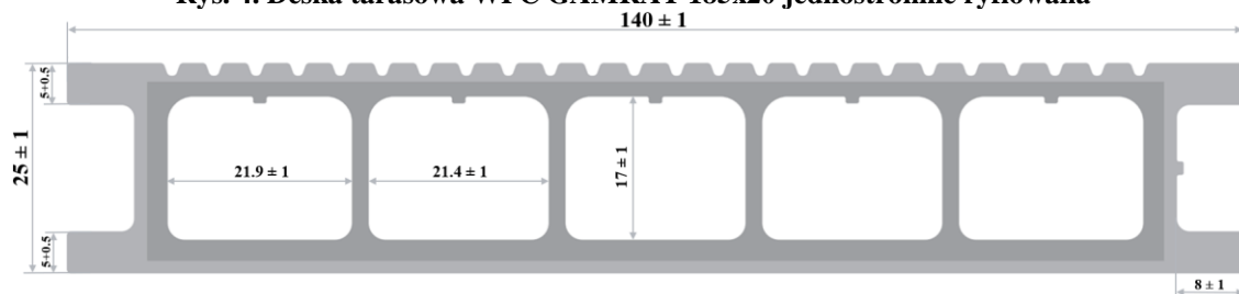
Rys. 5. Deska tarasowa WPC GAMRAT 140x25 SLIM jednostronnie ryflowana
