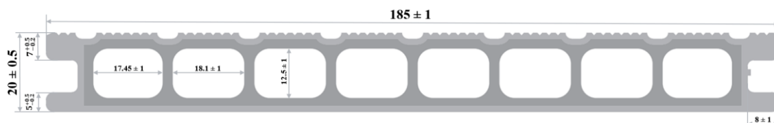
Rys. 4. Deska tarasowa WPC GAMRAT 185x20 jednostronnie ryflowana
