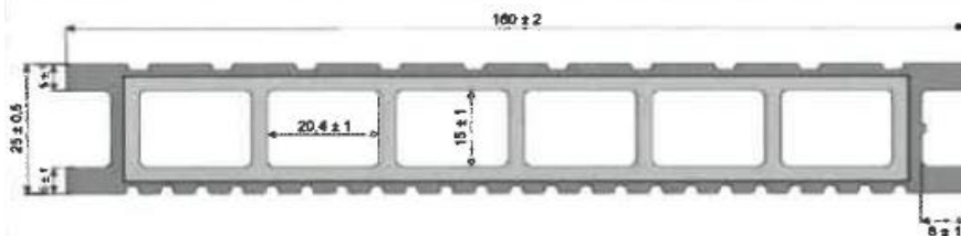
Rys. 1. Deska tarasowa WPC GAMRAT 160x25 dwustronnie ryflowana
