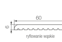
wymiary kompozytowej listwy wykończeniowej (mm)
