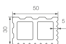
wymiary legara (mm)
