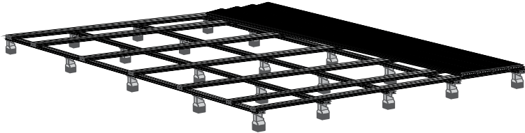
taras pływakowy na kratownicy metalowej położony na wspornikach poziomujących z tworzywa sztucznego
