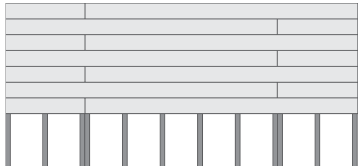
układ legarów przy czołowym połączeniu desek - taras na tzw. „mijankę”
