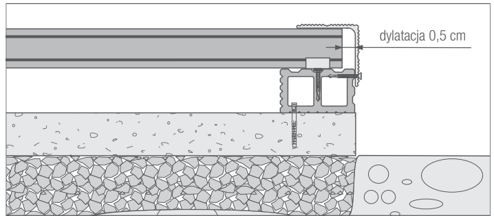
dylatacja 0,5 cm pomiędzy kompozytową listwą wykończeniową a czołową powierzchnią deski
