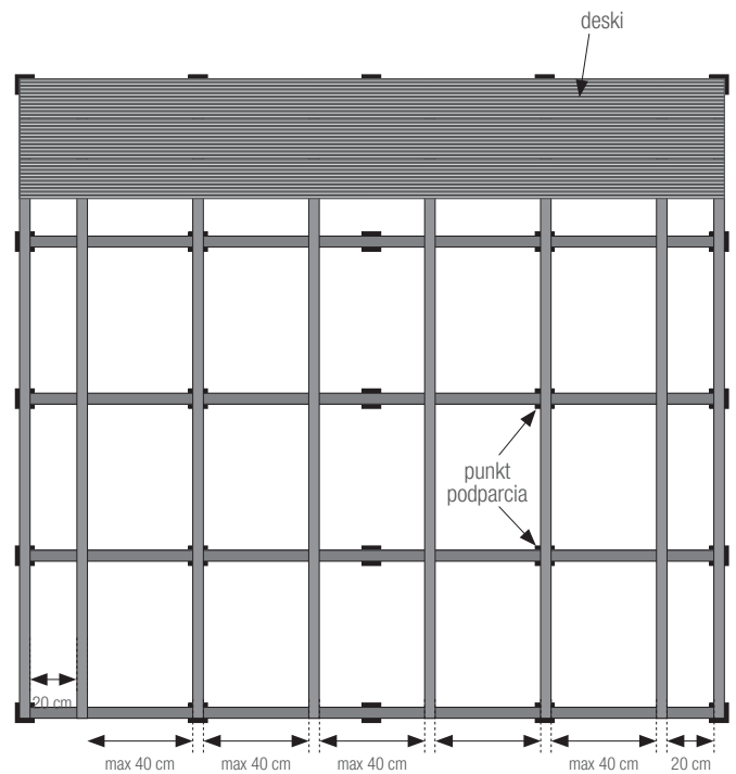
taras pływający na kratownicy metalowej rozstaw legarów
