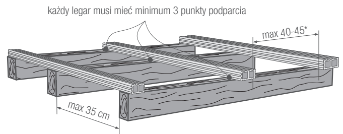
rozstaw legarów *40 cm - deska pełna *45 cm - deska komorowa
