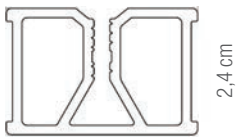
legar aluminiowy niski
