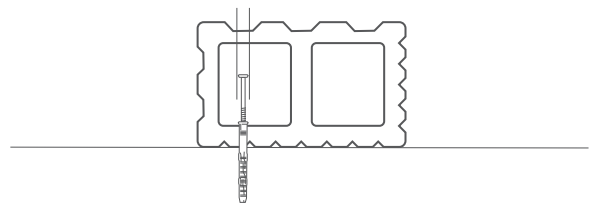
mocowanie legara w układzie poziomym
