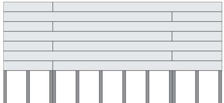
układ legarów przy czołowym połączeniu desek - taras na tzw. „miankę”
